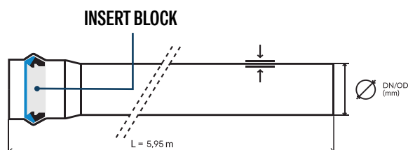
TUBO BIORIENTATO / ISO 16422 EN 17176 / PN25
